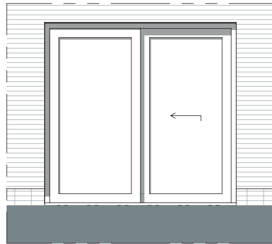
ACHTERGEVEL Schaal 1:50
