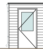
Rechtergevel bergingen 1:100
